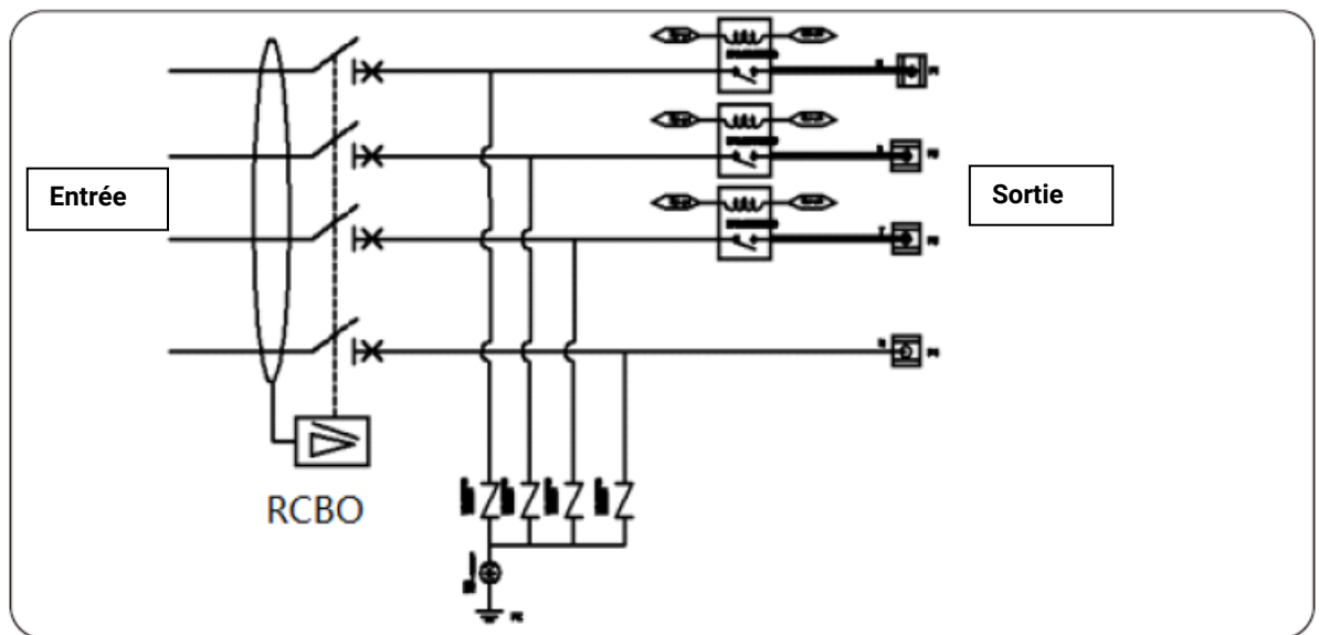
Fig J 1 - J . Schéma du circuit principal
